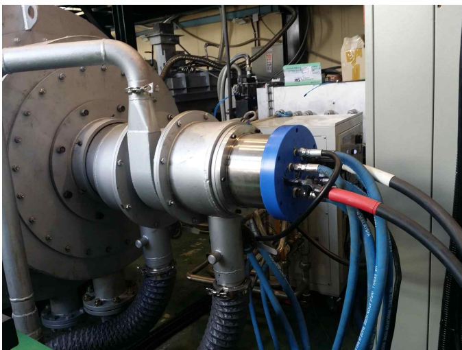
2-18. JS프라즈마-프라즈마 미분탄 혼소설비
