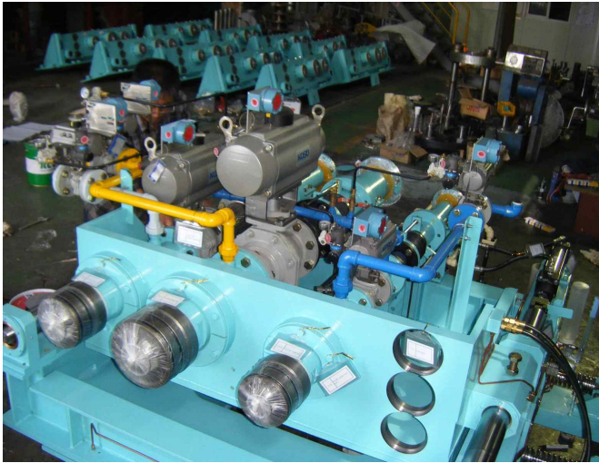
2-12. 포스칼슘-POSCO FOgas burner 및 열풍발생로
